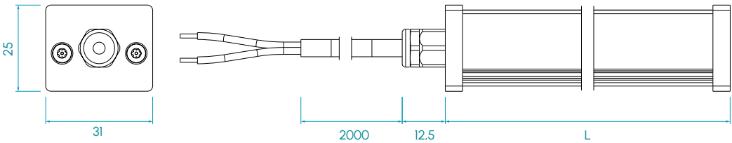
Versión axial
