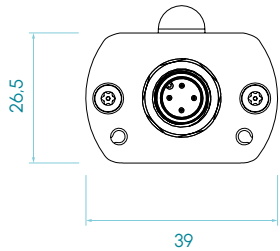
Sensor movimiento + entrada axial M12A
