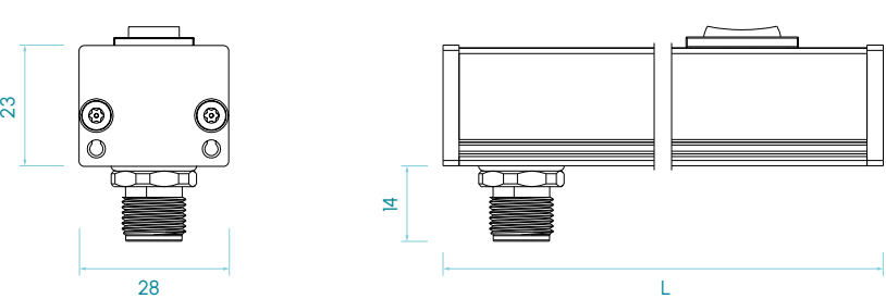
Interruptor + entrada radial M12A
