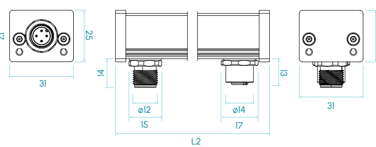
Versión radial M12A
