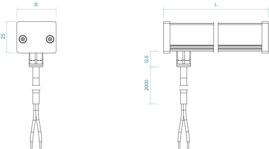
Versión radial
