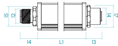
Versión axial M12A
