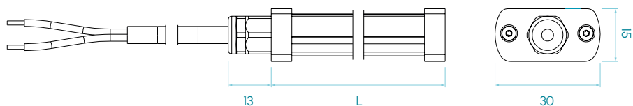
Versión axial M8A
