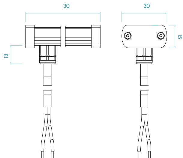
Versión radial M8A
